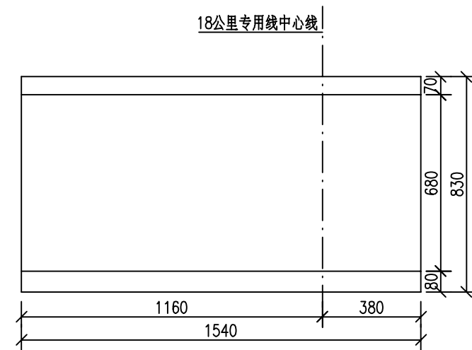
①#、②#箱体立面图
