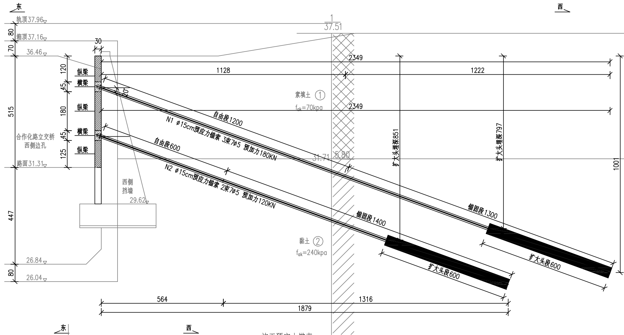
施工预应力锚索 施工步骤四
