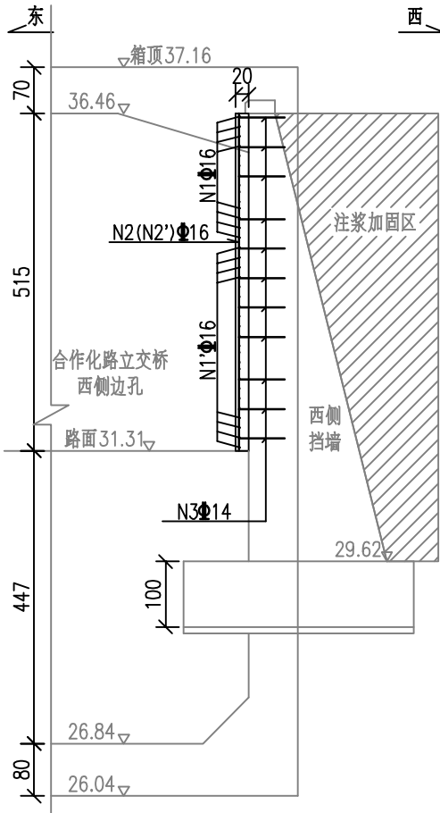
加固面板钢筋剖面布置图
