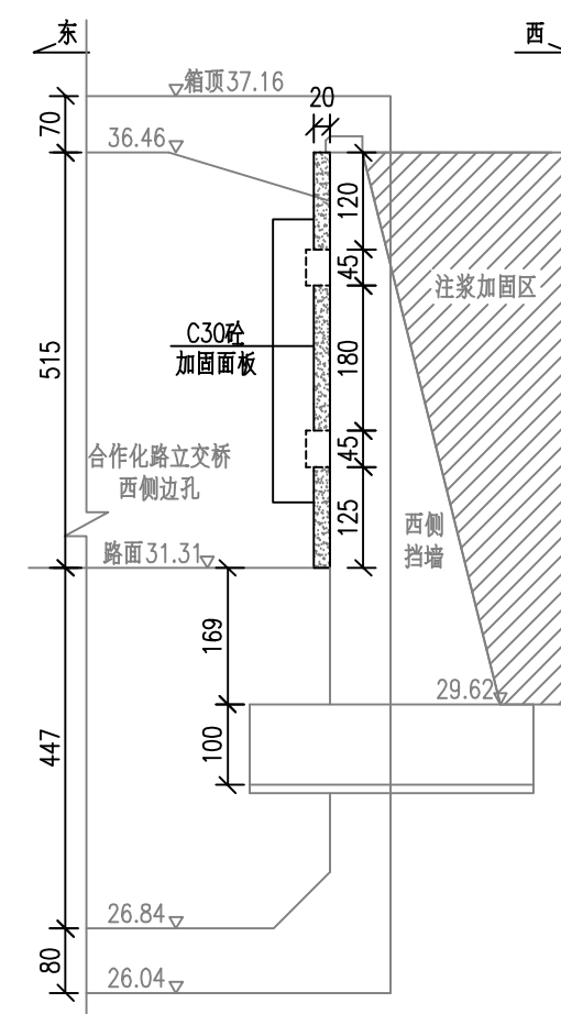
施工C30砼加固面板 (1-1) 施工步骤二 1:100
