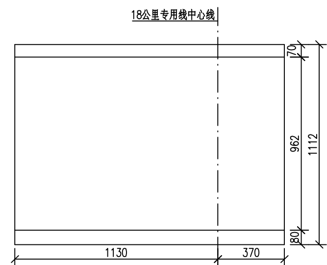
③#、④#箱体立面图
