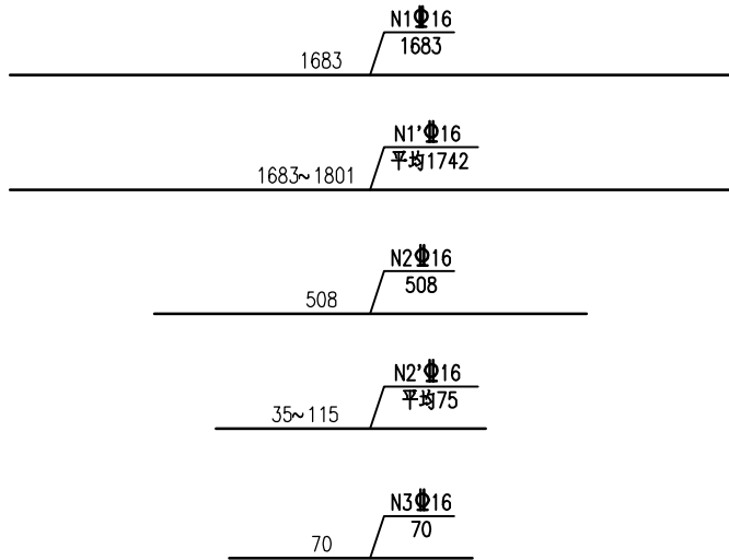
钢筋大样图
