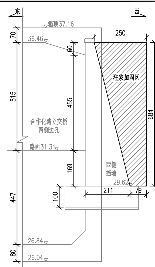
挡墙注浆加固剖面图 施工步骤一 1:100
