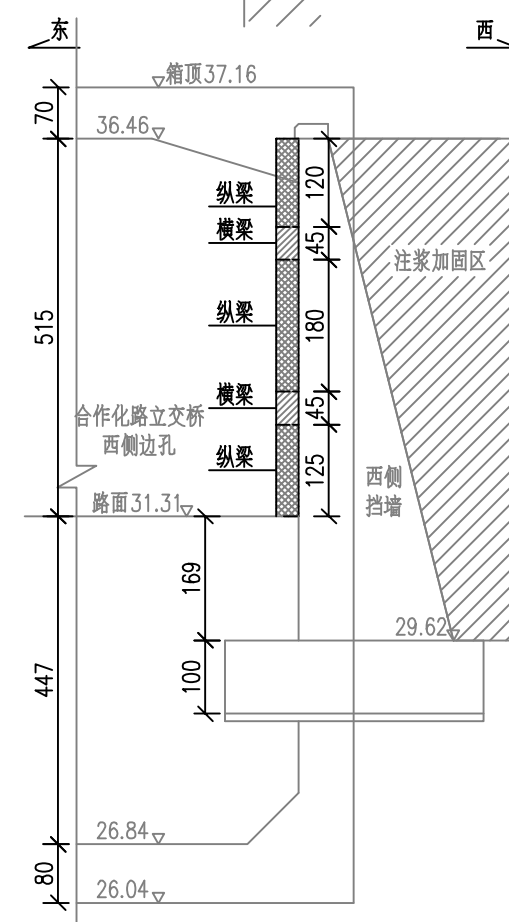
施工钢筋混凝土格构梁 (2-2) 施工步骤三 1:100
